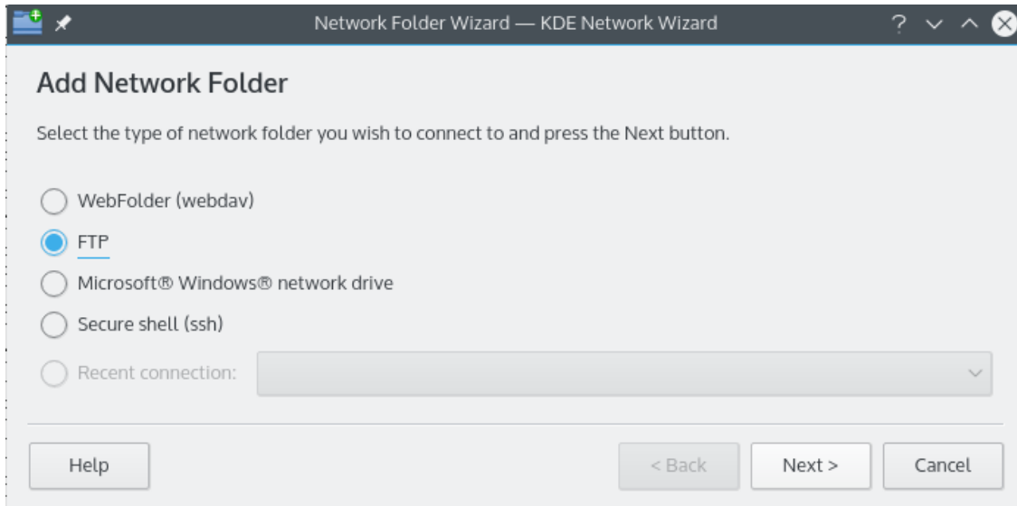
Nätverkskatalogguidens huvudfönster
