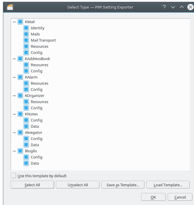
Auswahldialog
